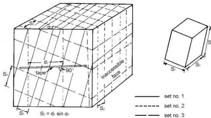
【그림 2.3.2】 노두 관찰을 통한 불연속면 간격 측정방법
